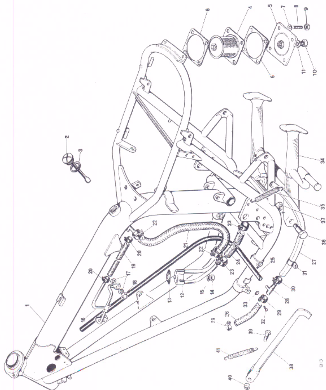
16. FRAME
