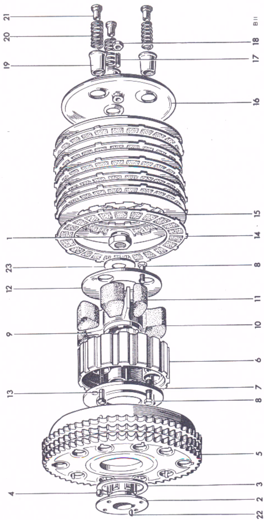
Fig. 14. CLUTCH
