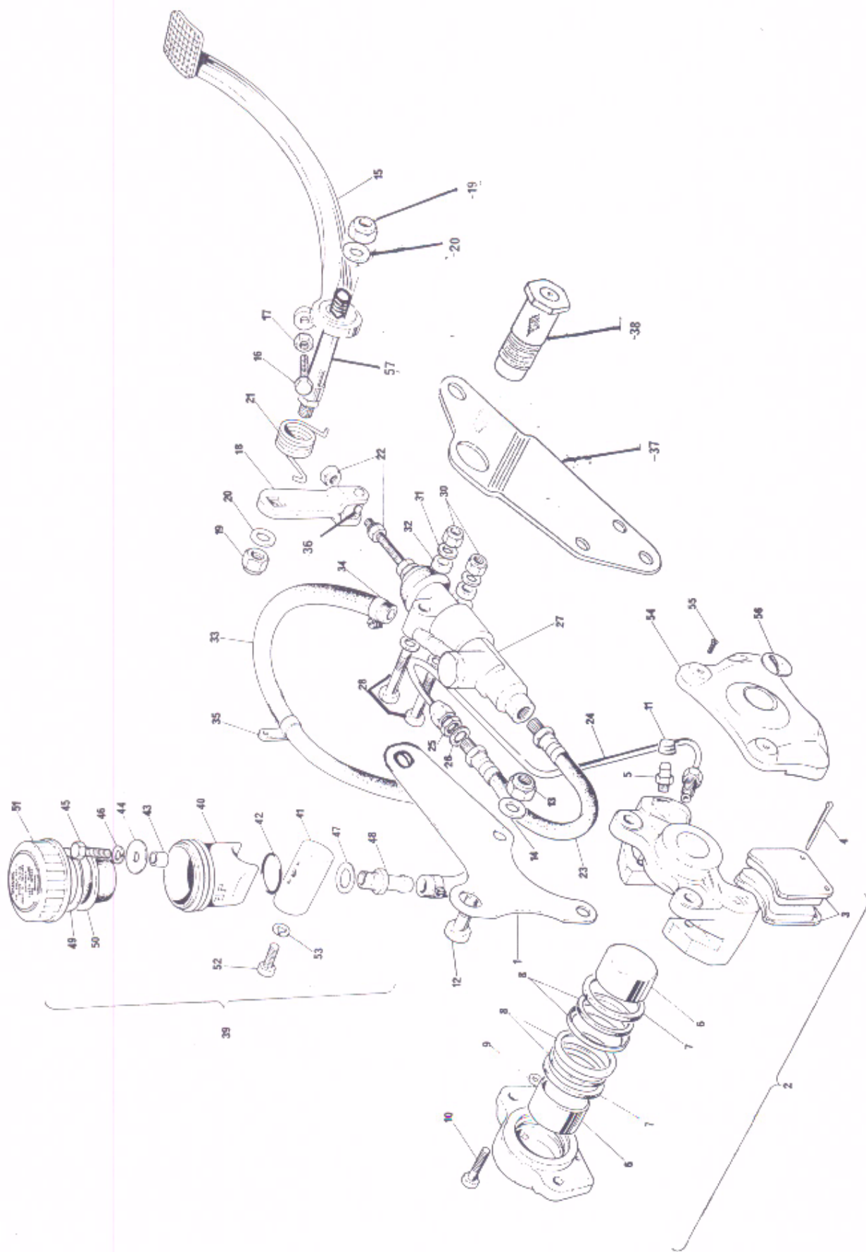
Fig. 25. REAR BRAKE
