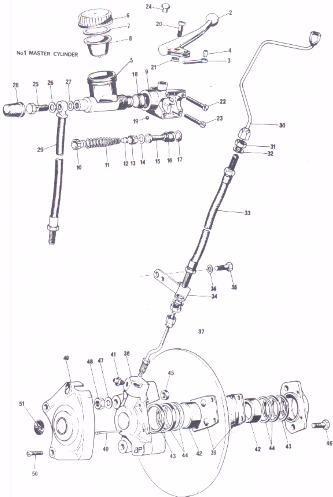
Fig. 23. FRONT BRAKE
