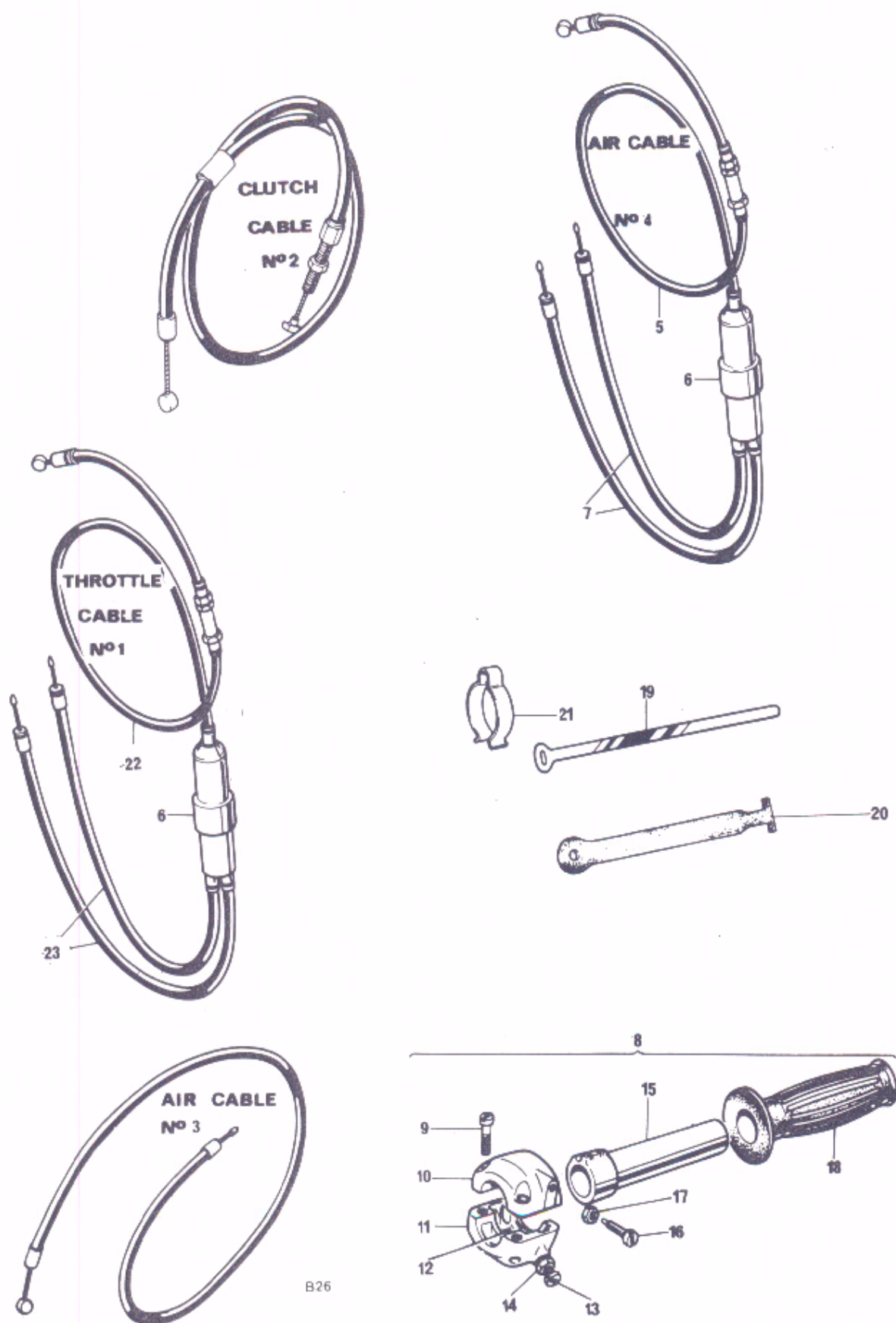
Fig. 30. CONTROL CABLES
